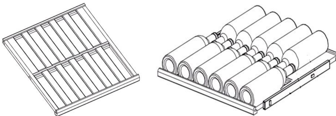
Выдвижная полка для DX-200.450K
