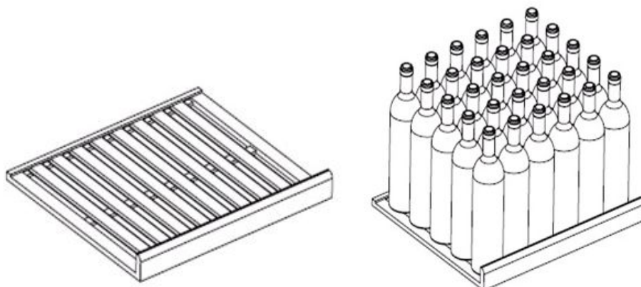
Стационарная полка для модели DX-114.270K (в целях безопасности крепится на болты к корпусу винного шкафа)
